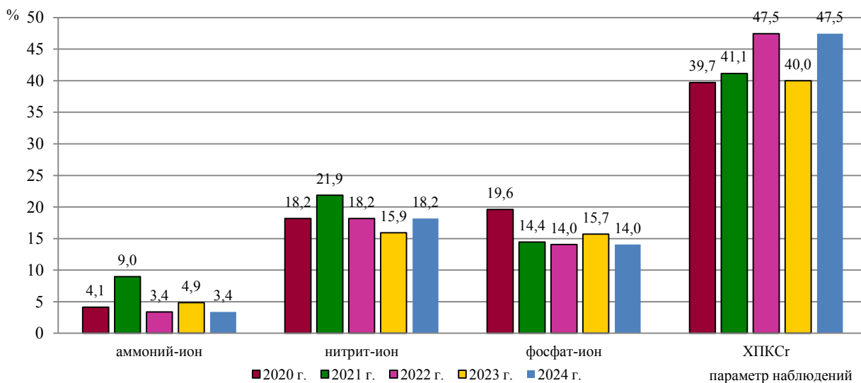
Рисунок 2.27 – Количество проб воды с повышенным содержанием химических веществ (в % от общего количества проб) в воде поверхностных водных объектов бассейна р. Неман за период 2020 – 2024 гг.
