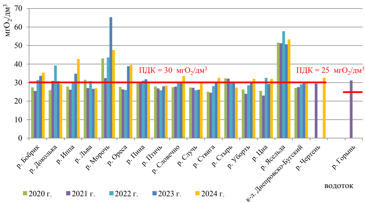
Рисунок 2.72 – Среднегодовые концентрации ХПК Cr в воде притоков р. Припять за 2020 – 2024 гг.
