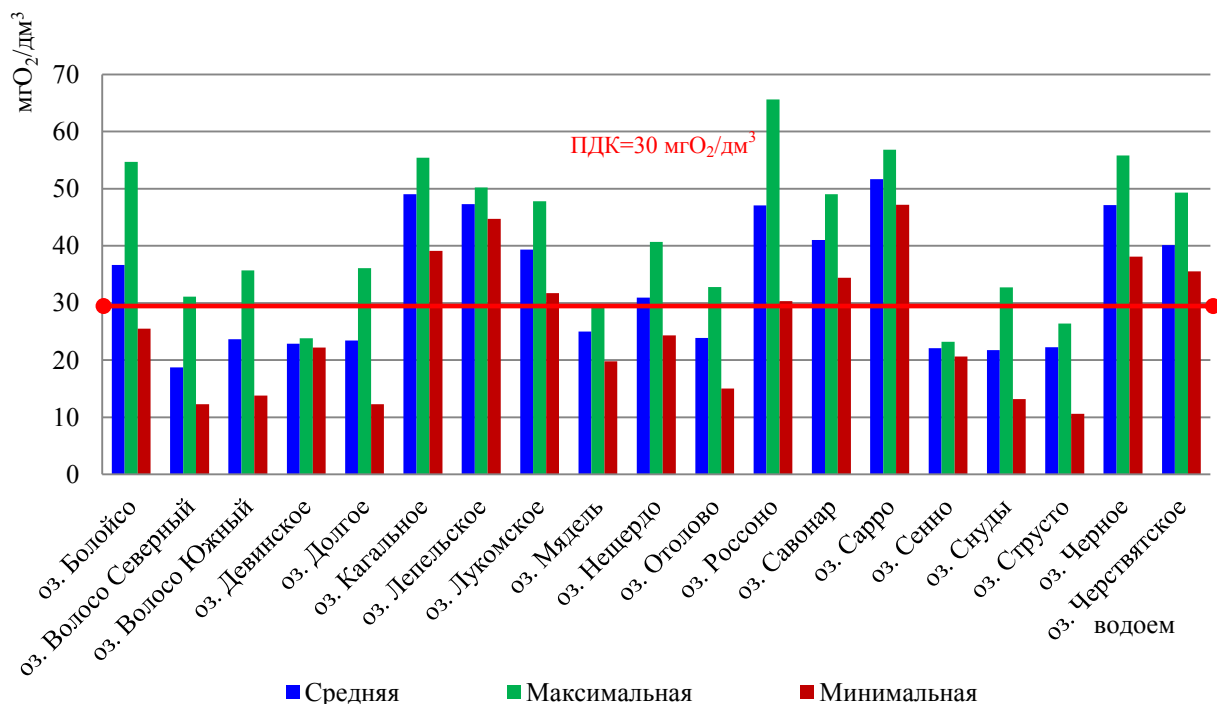
Рисунок 2.20 – Концентрация органических веществ по ХПК C t в воде водоёмов бассейна р. Западная Двина в 2024 г.
