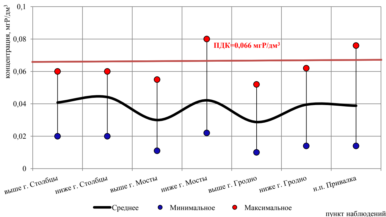
Рисунок 2.31 – Динамика концентраций фосфат-иона в воде р. Неман в 2024 г.
