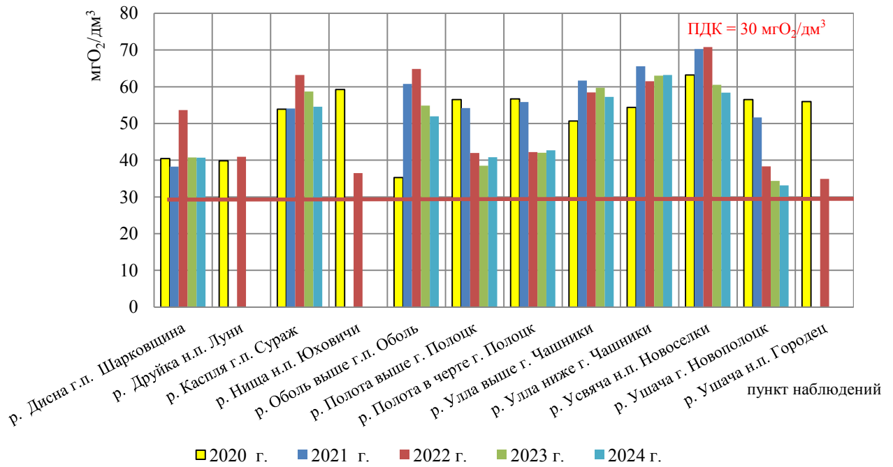
Рисунку 2.12 – Среднегодовые концентрации органических веществ, определяемые по ХПК Cr , в воде притоков р. Западная Двина за 2020 – 2024 гг.
