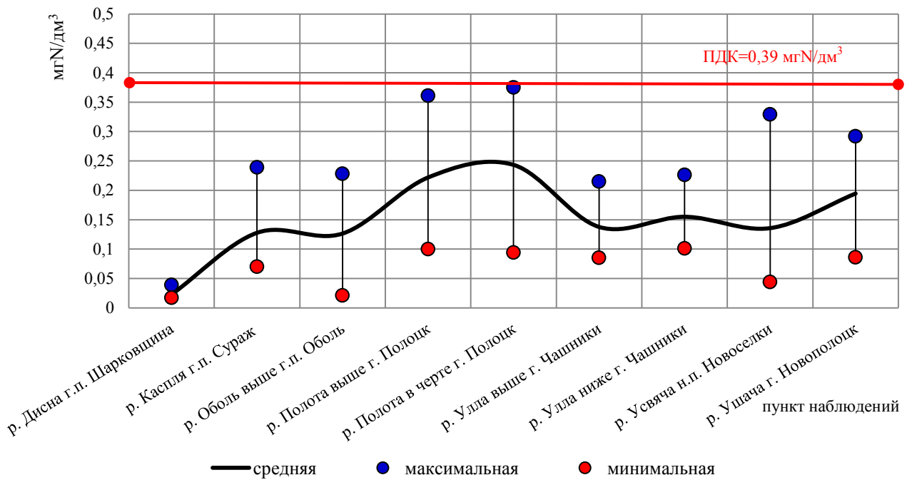
Рисунку 2.13 – Содержание аммоний-иона в воде притоков р. Западная Двина в 2024 г.
