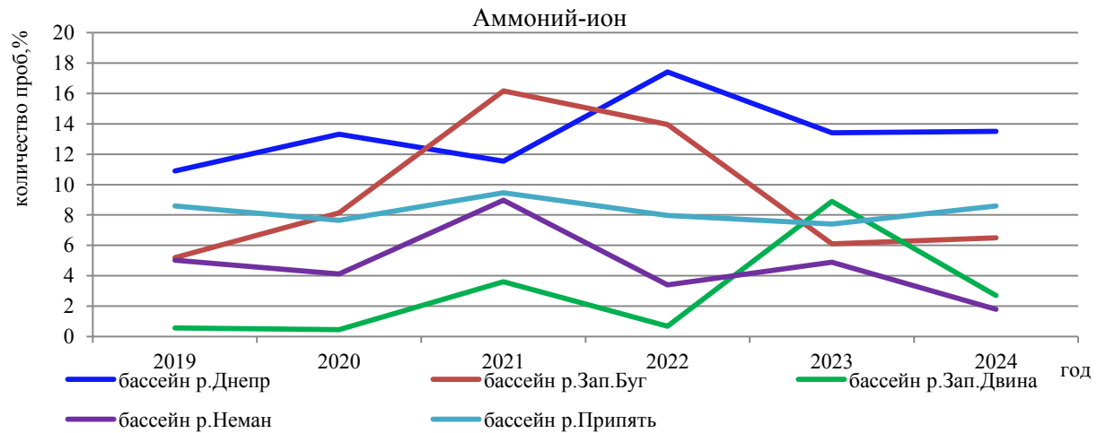
Рисунок 2.79 – Среднегодовые концентрации аммоний-иона, нитрит-иона, фосфат-иона, фосфора общего за период 2019 – 2024 гг.
