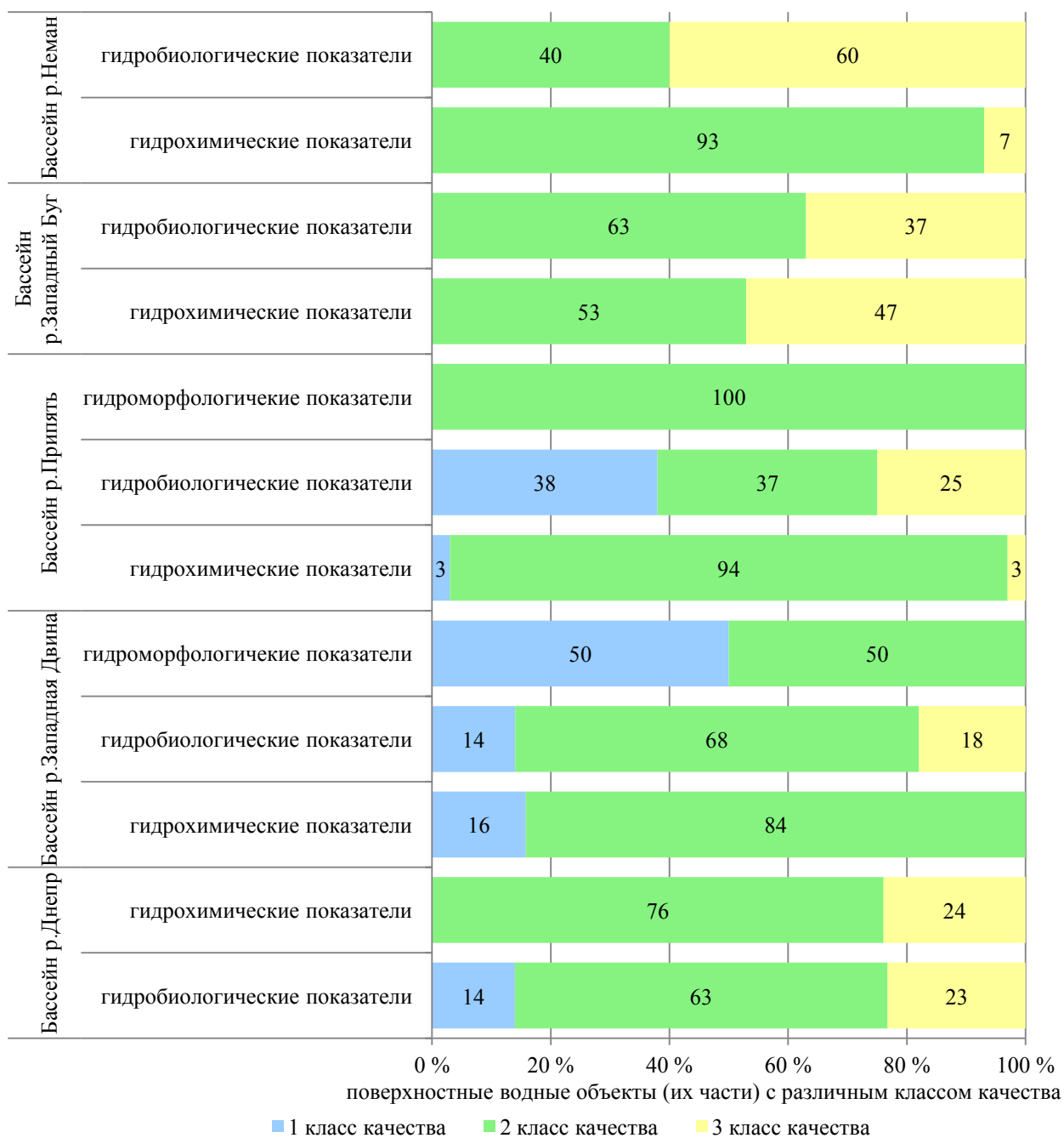
Рисунок 2.1 – Классы качества поверхностных водных объектов (их частей) по гидробиологическим, гидрохимическим и гидроморфологическим показателям в 2024 г.
