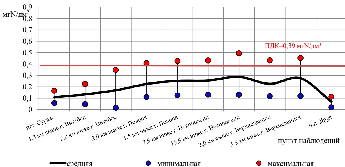
Рисунок 2.7 – Содержание аммоний-иона в воде р. Западная Двина в 2024 г.
