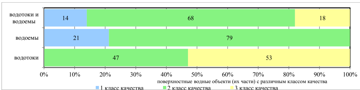
Рисунок 2.3 – Относительное количество поверхностных водных объектов (их частей) бассейна р. Западная Двина с различными классами качества по гидробиологическим показателям в 2024 г.
